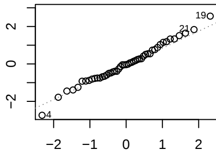
Normal Q-Q
