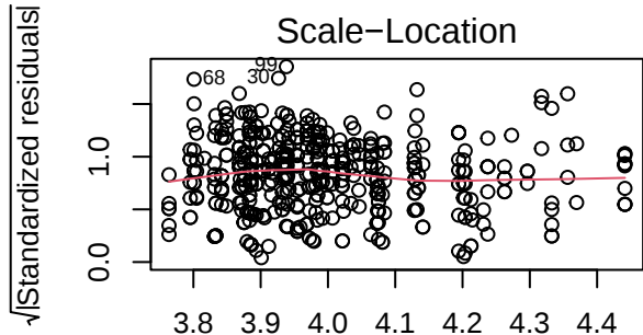
Fitted values
