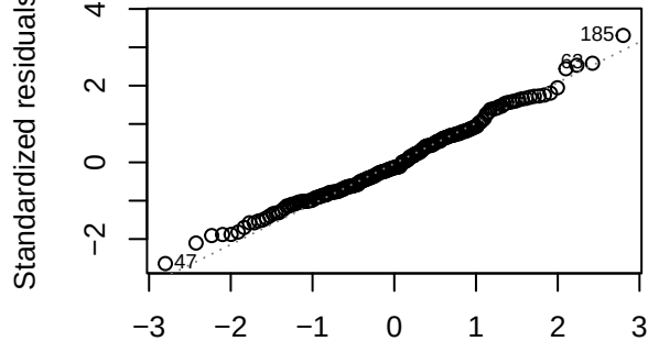
Normal Q-Q
