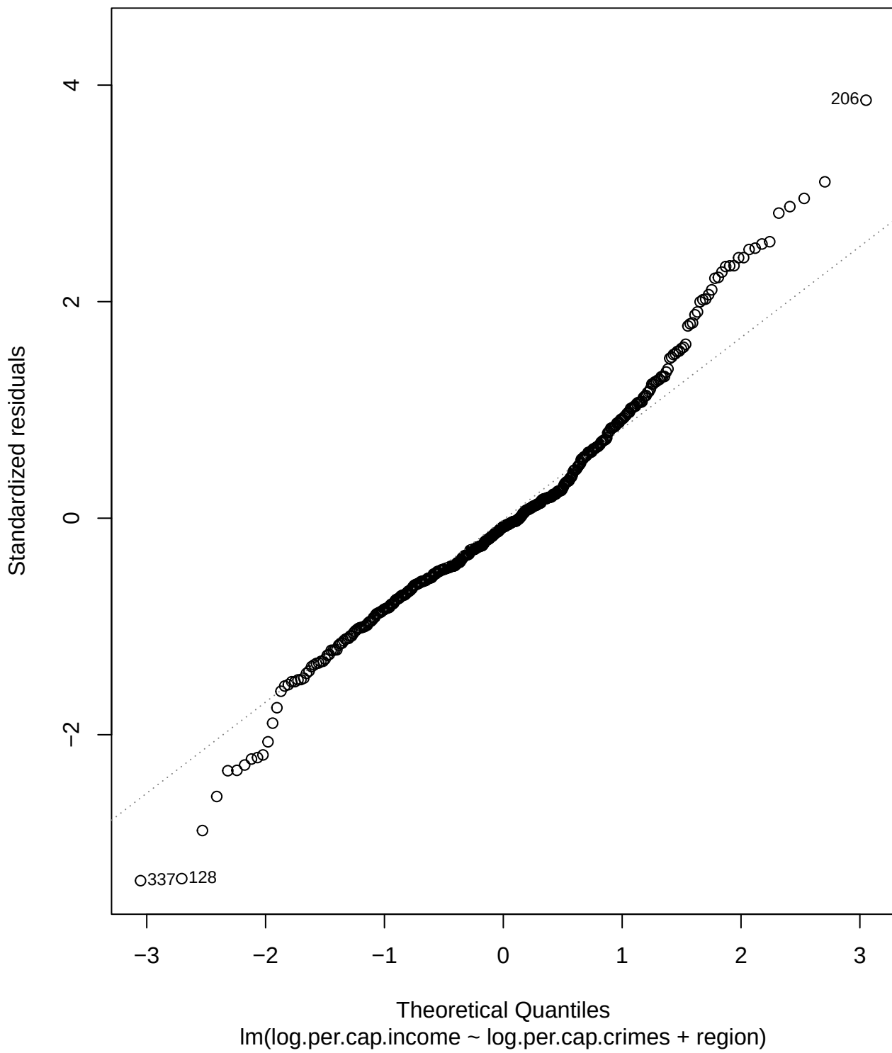
Normal Q-Q
