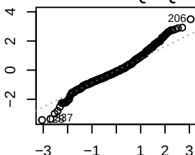
Normal Q-Q
