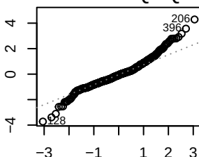
Normal O-O
