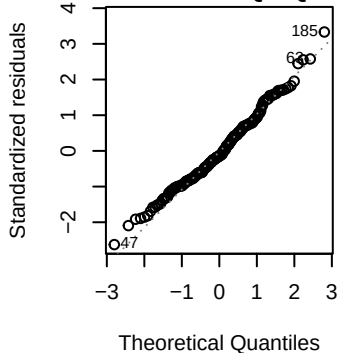
Normal Q-Q
